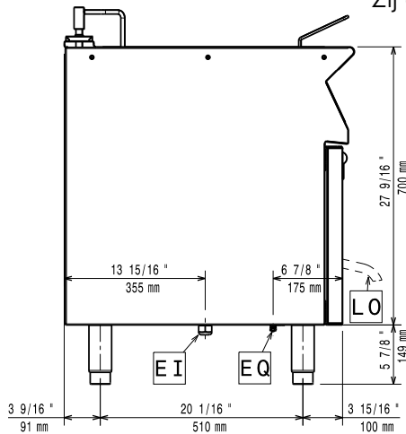
Zij aanzicht
