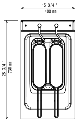
Boven aanzicht
